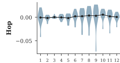
Base GPT-2
