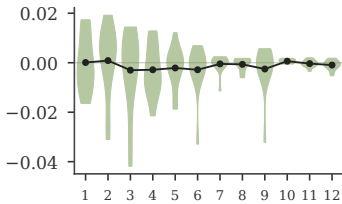
Kallini
